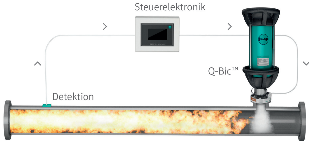
Schematische Darstellung einer Löschmittelsperre.
